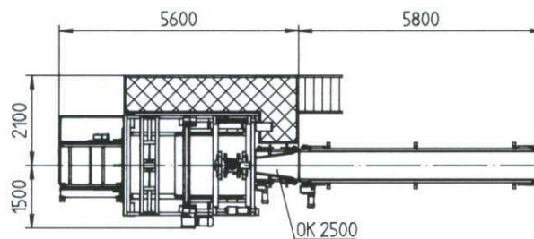
Draufsicht PIKOMAT HDQ-Kompakt
