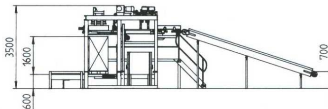
Seitenansicht PIKOMAT HDQ-Kompakt
