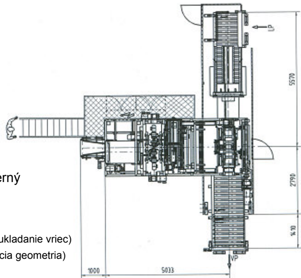
Príklad zostavy pre PIKOMAT-HDQ HD
