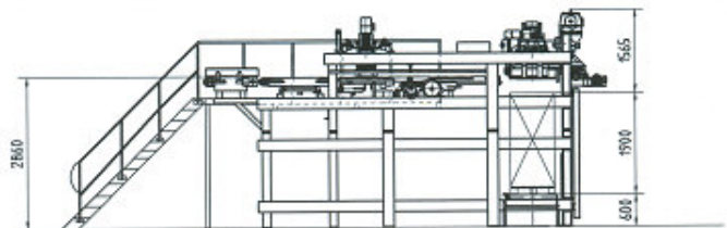
Otočné zariadenie PIKOMAT-HDQ HD
