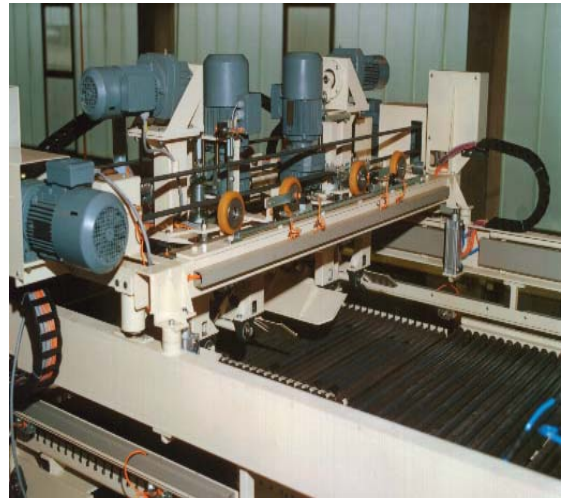
Otočné zariadenie PIKOMAT-HDQ HD
