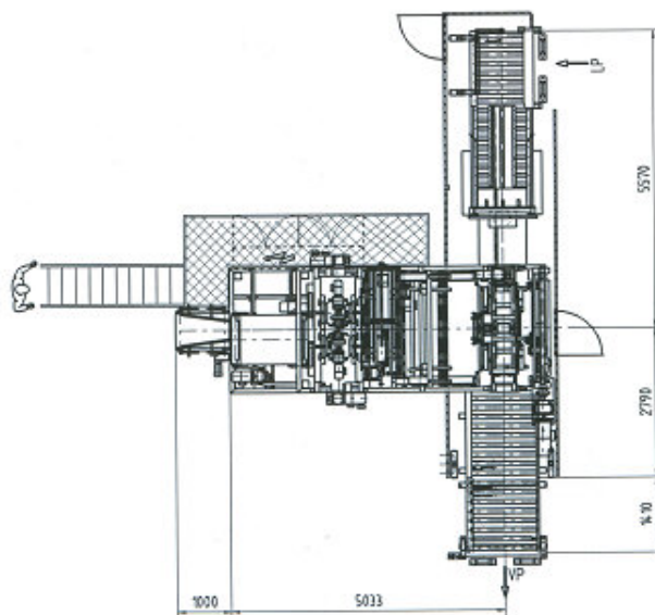
Пример установки PIKOMAT-HDQ HD
