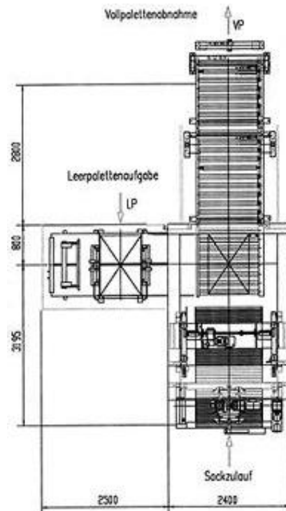
Примерная схема PIKOMAT NDL-Portal
