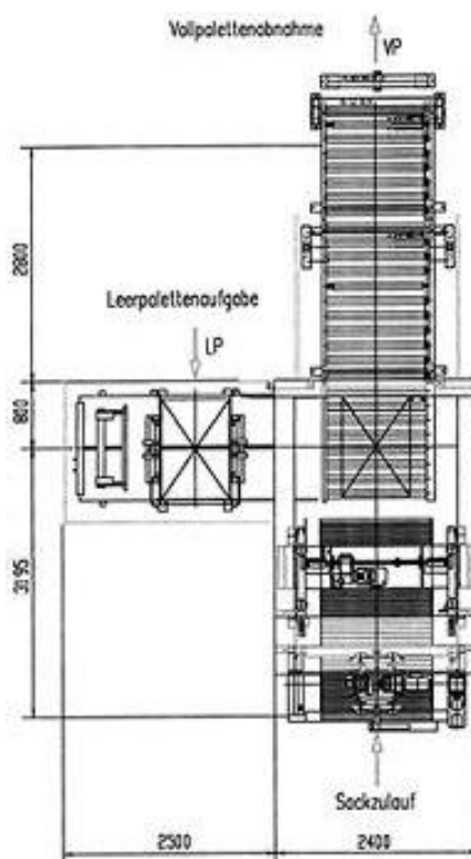
Exemplo de instalação do PIKOMAT NDL-pórtico
