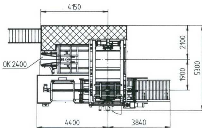
Draufsicht PIKOMAT HPS-Sackpalettierer
