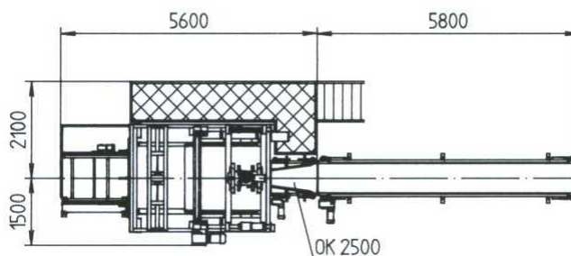
Draufsicht PIKOMAT HDQ-Kompakt
