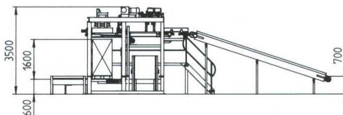
Seitenansicht PIKOMAT HDQ-Kompakt
