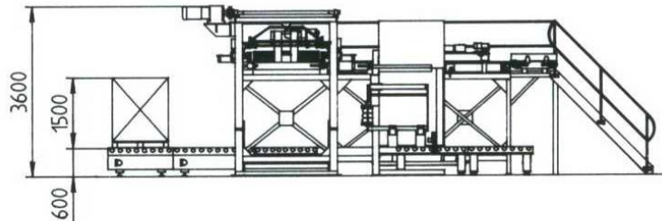
Seitenansicht PIKOMAT HPS-H-Sackpalettierer
