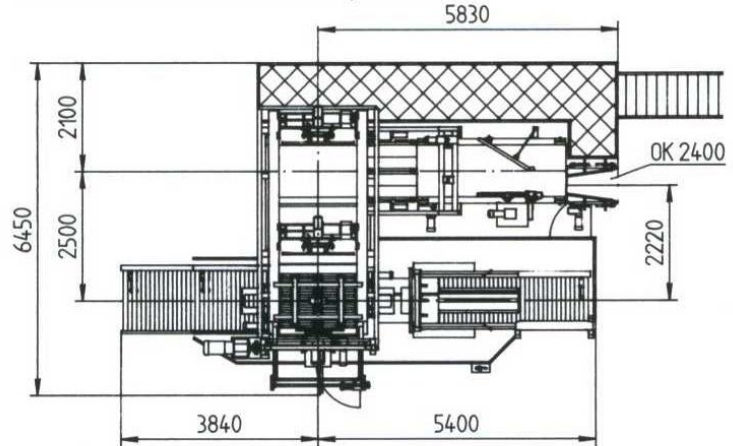
Draufsicht PIKOMAT HPS-H-Sackpalettierer
