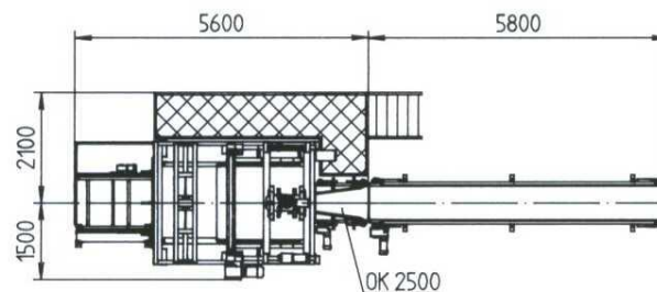
Vista aerea PIKOMAT HDQ-Kompakt
