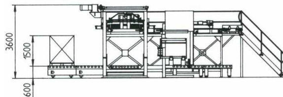
Vista lateral PIKOMAT-HPS-H-Paletizador de sacos
