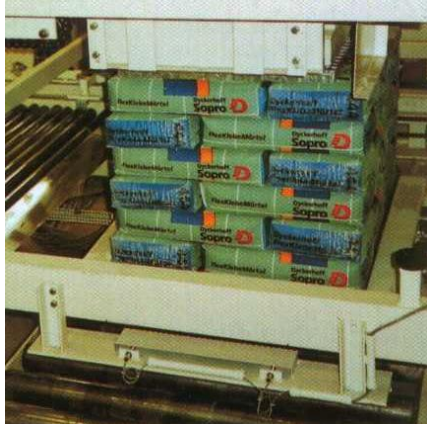
Ilustraciòn de apilado PIKOMAT HPS-H-Paletizador de sacos
