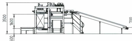
Ilustraciòn de apilado PIKOMAT HDQ - Compacto
