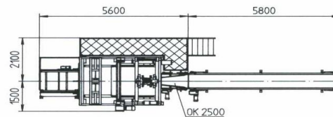
Vista lateral PIKOMAT HDQ - Compacto
