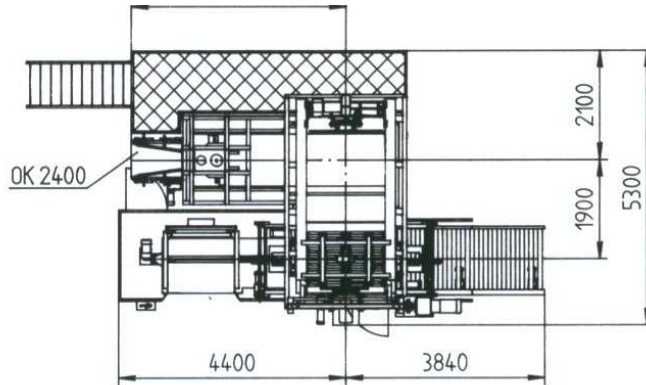
Draufsicht PIKOMAT HPS-Sackpalettierer
