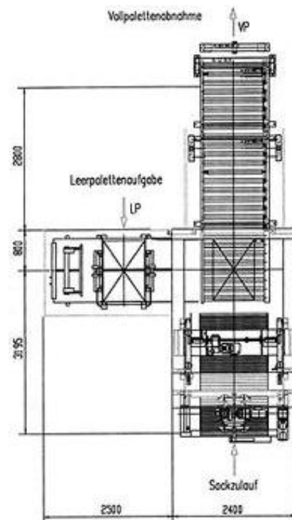
Aufstellungsbeispiel PIKOMAT NDL-Portal
