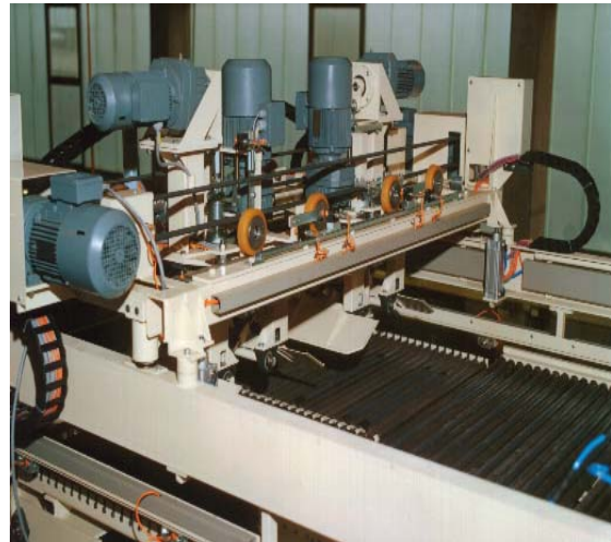
Drehstern PIKOMAT-HDQ HD
