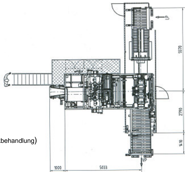
Aufstellungsbeispiel PIKOMAT-HDQ HD
