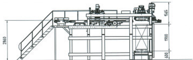
Drehstern PIKOMAT-HDQ HD
