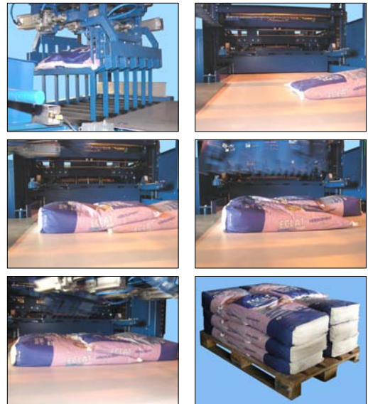
Abb. Stapelbild im 4er-Verband, überlappt
