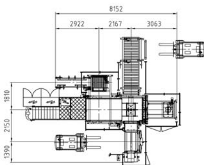
Abb. Einbaubeispiel HDQ – Kompakt - Greifsystem
