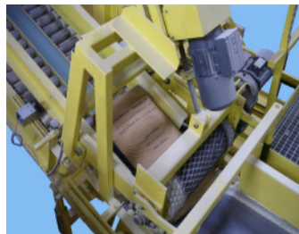
Staurollenbahn
